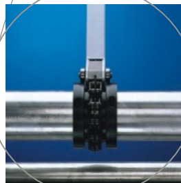
Fácil colocación de la cadena de corte de varios piñones y del MRA mediante las mordazas
